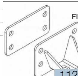
MORSETTO DI FISSAGGIO LONGITUDINALE
