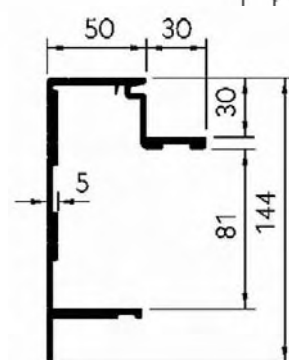
STRUTTURA PERIMETRALE da fissare sulle traverse del telaio
