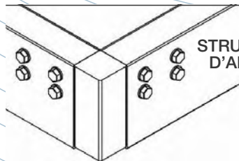
MORSETTO DI FISSAGGIO TRASVERSALE
