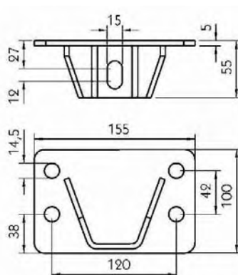
STAFFA DI FISSAGGIO BOX per veicoli fino a 12 t
