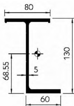
STRUTTURA SECONDARIA da fissare sui longheroni del veicolo
