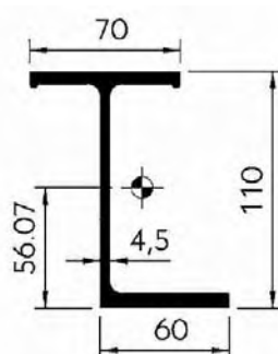
STRUTTURA SECONDARIA da fissare sui longheroni del veicolo
