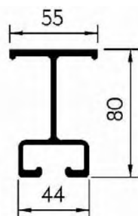
TRAVERSE DEL TELAIO da fissare sulla struttura secondaria
