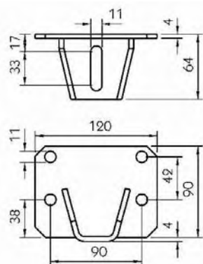
STAFFA DI FISSAGGIO BOX per veicoli fino a 3,5 t
